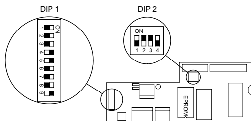
Местоположение переключателей DIP 1 и DIP 2 на микропроцессоре PFU 2000
