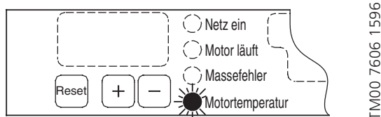
Рис. 27. Индикация температуры электродвигателя на блоке защиты CU 3.
