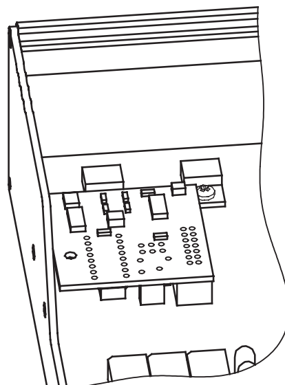
Рис. 49. Правильное сочленение модуля связи RS-485 со штепсельным разъемом JP106
