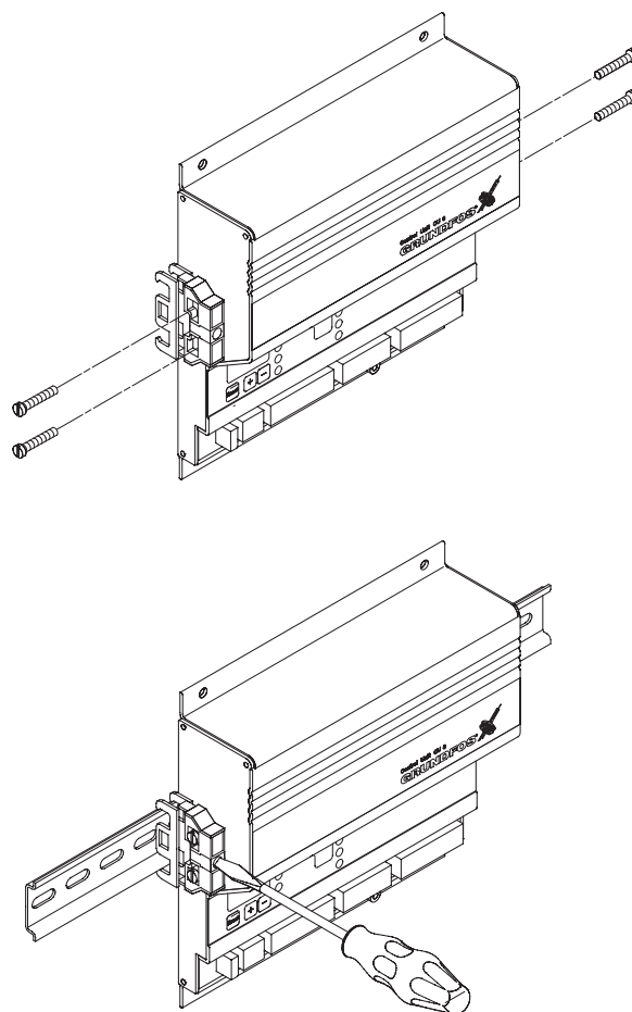
Рис. 4. Монтаж блока защиты CU 3 на направляющем рельсе.
