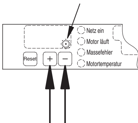
Рис. 23. Клавиши "+" и "-" блока защиты CU 3.
