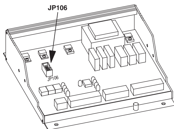
Рис. 48. Стыковка модуля связи RS-485 со штепсельным разъемом JP106.
