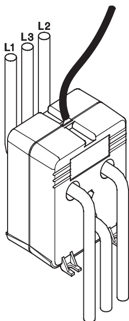
Рис. 45. Обеспечение правильной последовательности чередования фаз.
