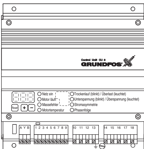
Рис. 1. Общий вид блока защиты CU 3.
