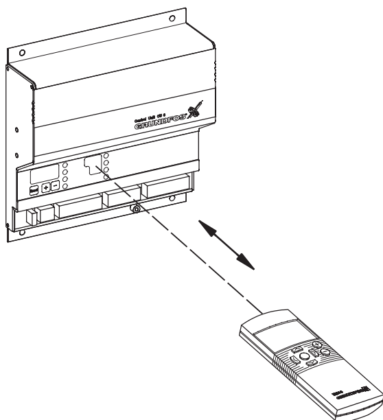
Рис. 35. Визуальный контакт между блоком защиты CU 3 и ПДУ R100.
