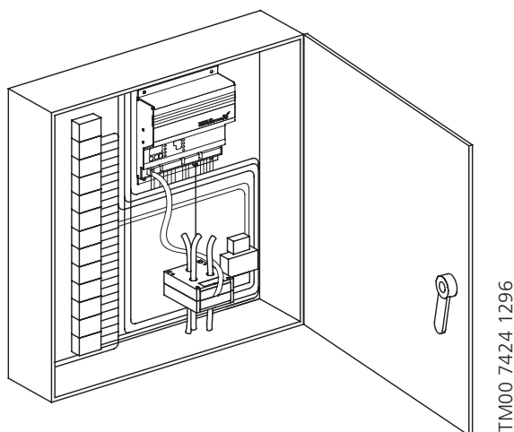
Рис. 3. Монтаж блока защиты CU 3 на монтажной плате.
