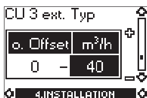
Рис. 10. Выбор типа датчика, подключенного к блоку защиты CU 3 через клеммы 1, 2 и 3.
