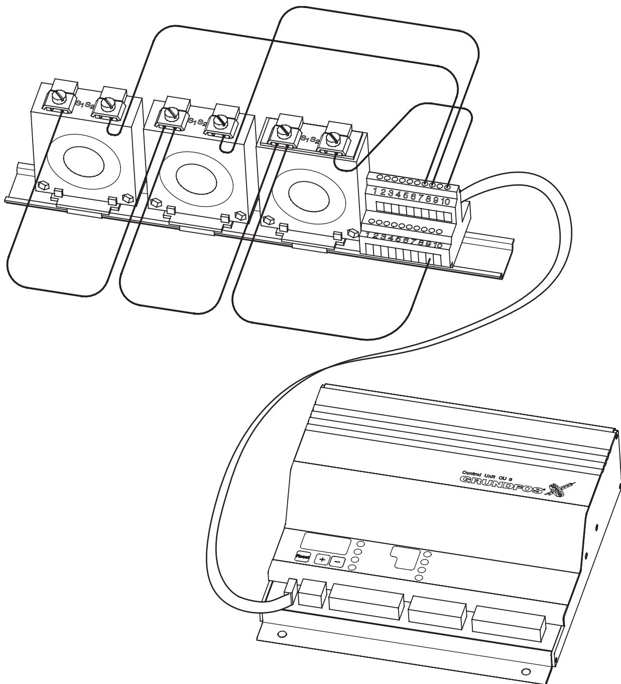
Рис. 8. Применение у электродвигателей без температурных датчиков отдельных преобразователей сигналов вместо одного преобразователя.
