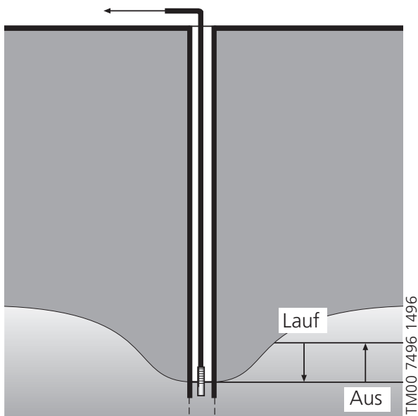
Рис. 44. Соотношение времени работы и отключения насоса при резко пониженном уровне грунтовых вод.
