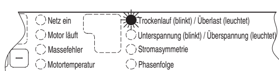
Рис. 29. Индикация перегрузки на блоке защиты CU 3.
