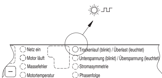
Рис. 28. Индикация сухого хода на блоке защиты CU 3.
