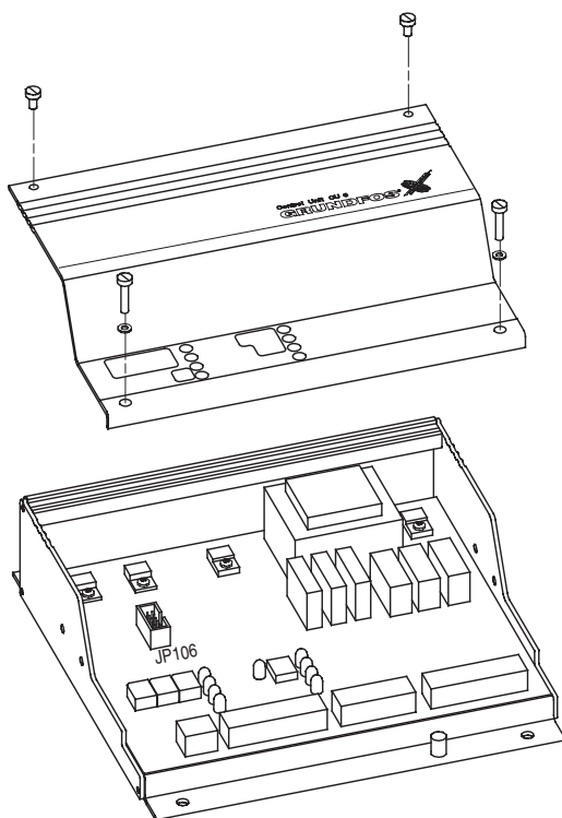
Рис. 47. Монтаж модуля связи RS-485.
