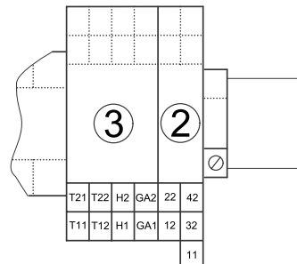
Рис. 15 Клеммы
