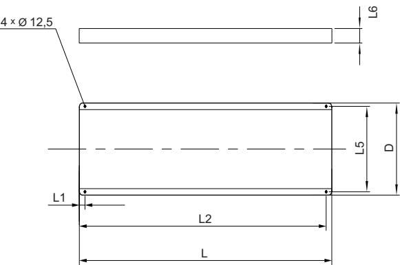
Шкаф управления. Для исполнения В
