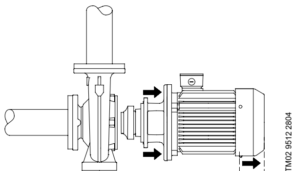
Рис. 1 Демонтаж электродвигателя
