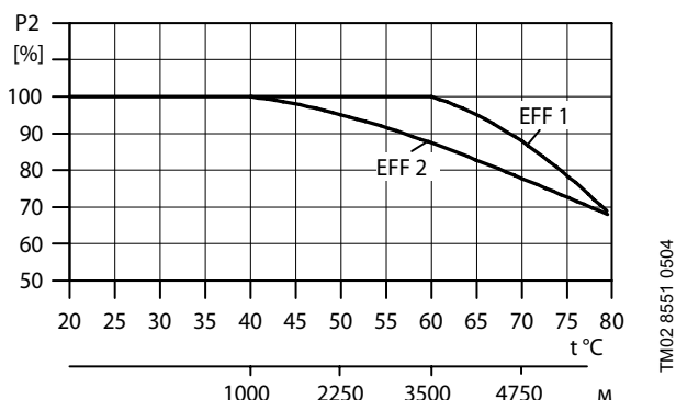
Рис. 8 Зависимость мощности электродвигателя P2 от температуры/высоты над уровнем моря
