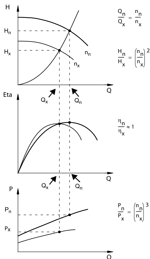
Рис. 12 Уравнения подобия
