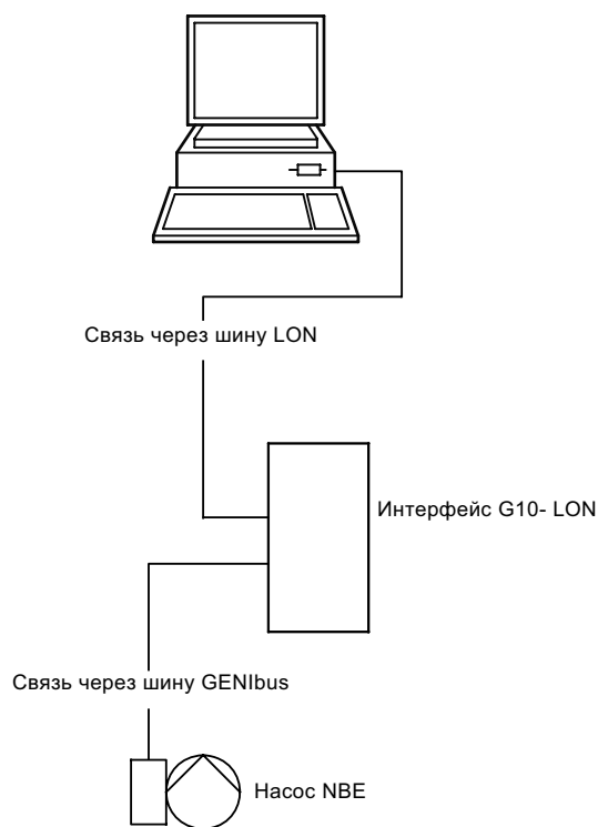
Рис. 13 Структура системы диспетчеризации
