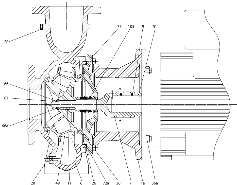
Рис. 5 Чертёж в разрезе насоса NB
