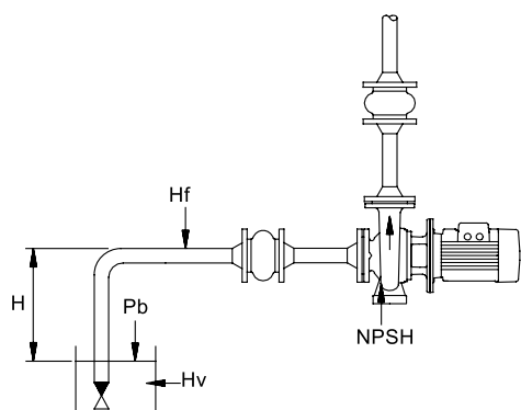
Рис. 9 Схема открытой системы с насосом NB
