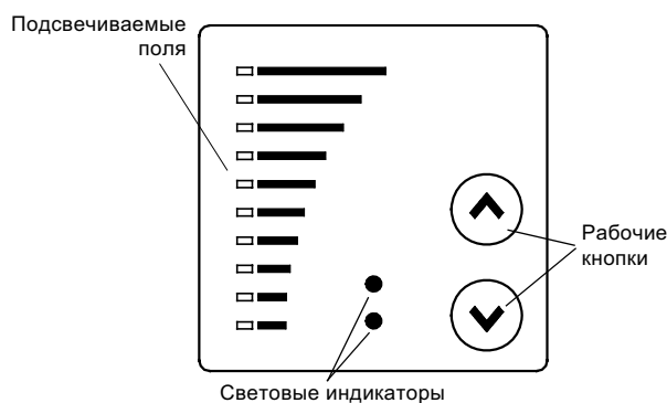
Рис. 15 Панель управления насоса NBE
