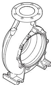
Рис. 6 Корпус насоса
