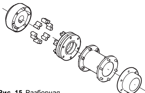
Рис. 15 Разборная
